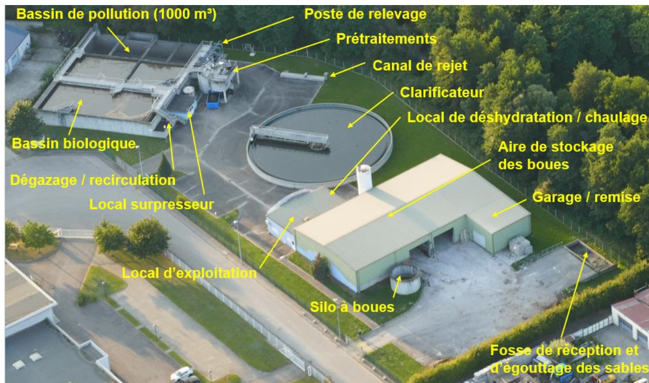
Vue aérienne des différents ouvrages de la station d'épuration de Niedermodern
